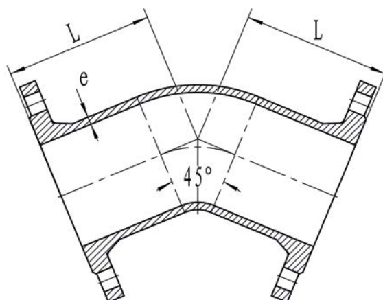
COUDE DOUBLE BRIDE 45° (1/8)
