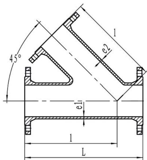
TE À BRIDES SORTIE 45°
